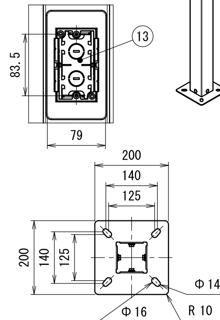
C拡大図 1/5
