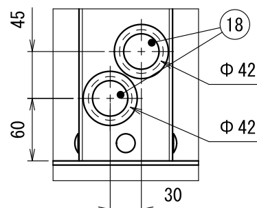
裏面底部拡大図 1/5
